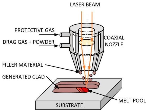
Figura 1: Princípio do funcionamento DMD
