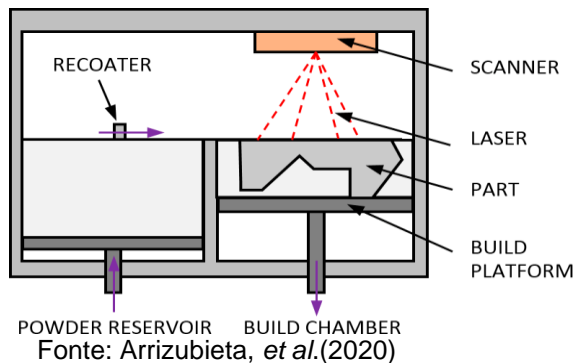
Figura 2: Princípio do funcionamento SLM
