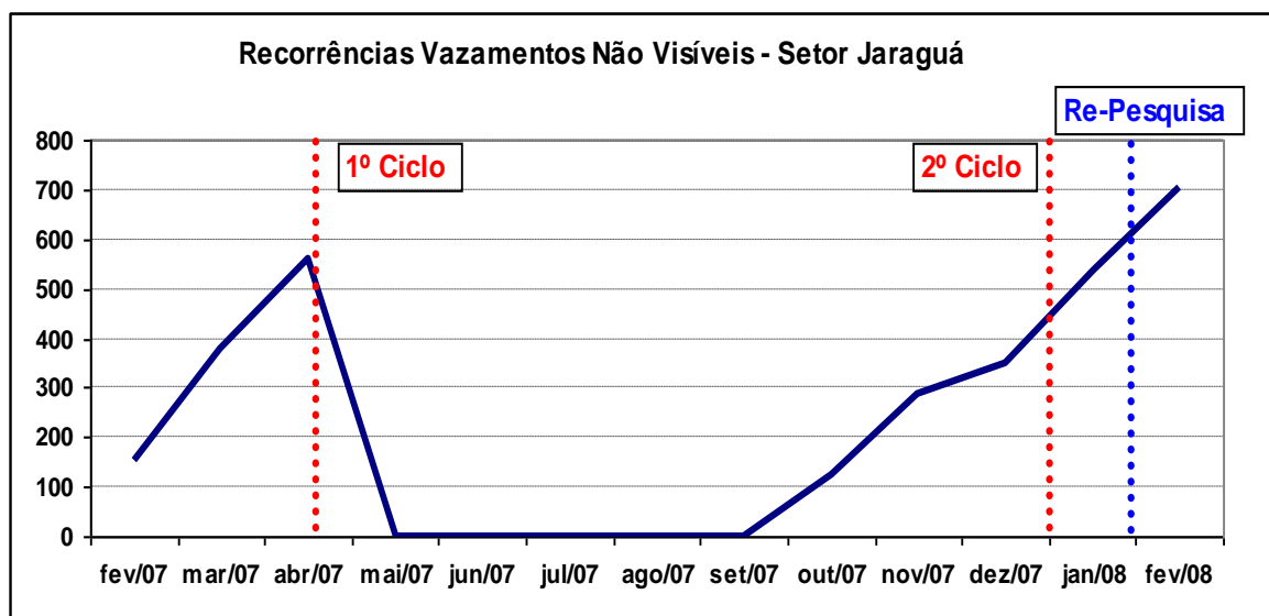
Figura 07 – Gráfico de Recorrência de Vazamentos no Setor Jaraguá (Fonte: Sabesp-MNEP/08)
