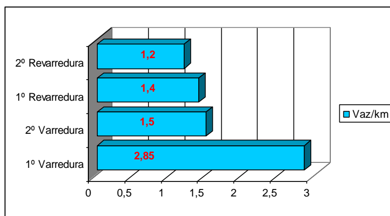
Figura 06 – Vazamentos por quilometro entre os Ciclos de Pesquisas no Setor Jaraguá (Fonte: Sabesp-MNEP/08)
